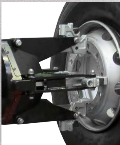
AUTO-CENTREUR UNIVERSEL 4 GRIFFES
